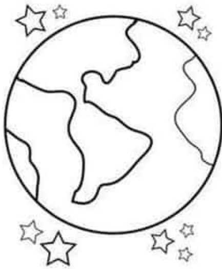
Earth
